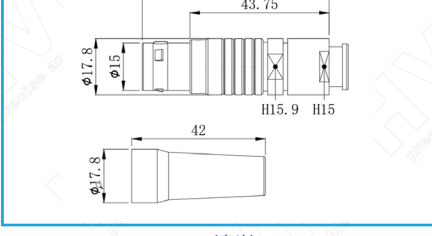
FGG(直头)
