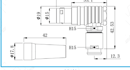
FHG(弯头)
